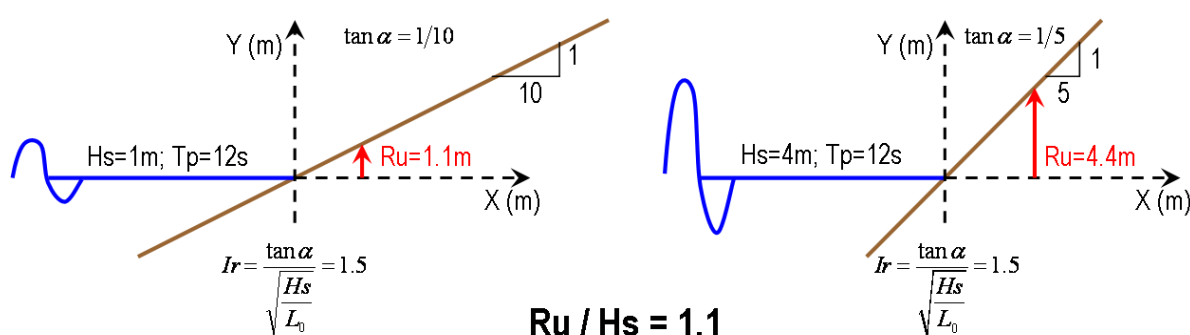
Figura 10. Ejemplo de dos perfiles con el mismo número de Iribarren ( Ir ) y run-up adimensional ( Ru/H_s ). Perfil izquierda: Pendiente 1/10, Ru = 1.1 m, H_s = 1 m, T_p = 12 s. Perfil derecha: Pendiente 1/5, Ru = 4.4 m, H_s = 4 m, T_p = 12 s
