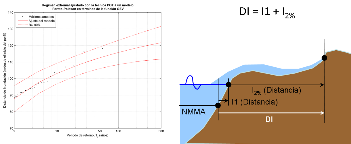
Figura 18. Ejemplo de ajuste del régimen extremal de distancia de inundación con nivel del mar y oleaje.
