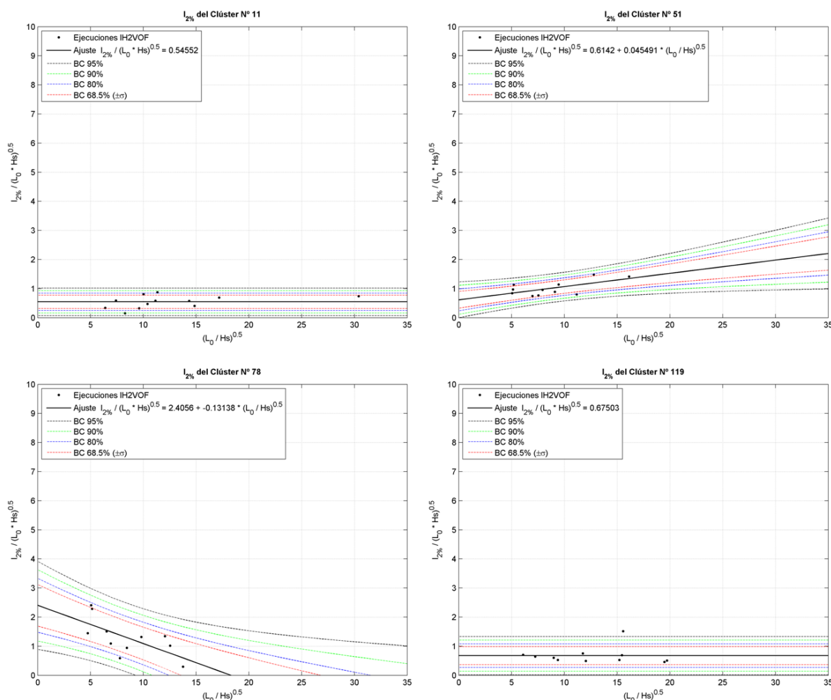
Figura 16. Ajustes lineales del alcance de la inundación adimensional ( I_{2\%}/\sqrt{L_0 H_s} ) en 4 clústers (Nº 11, 51, 78 y 119). Los puntos negros son los resultados de las ejecuciones del modelo IH-2VOF, la línea negra es el ajuste de los datos a una recta y las líneas discontinuas son distintas bandas de confianza al 95%, 90%, 80% y 68.5% respectivamente.
