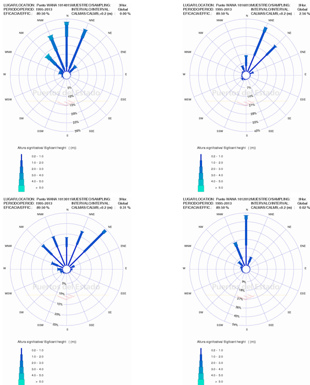
Figura 6. Oleaje en Tenerife (de arriba abajo y de izquierda a derecha: zona norte, este, sur, y oeste de la Isla de Tenerife). Fuente: Puertos del Estado
