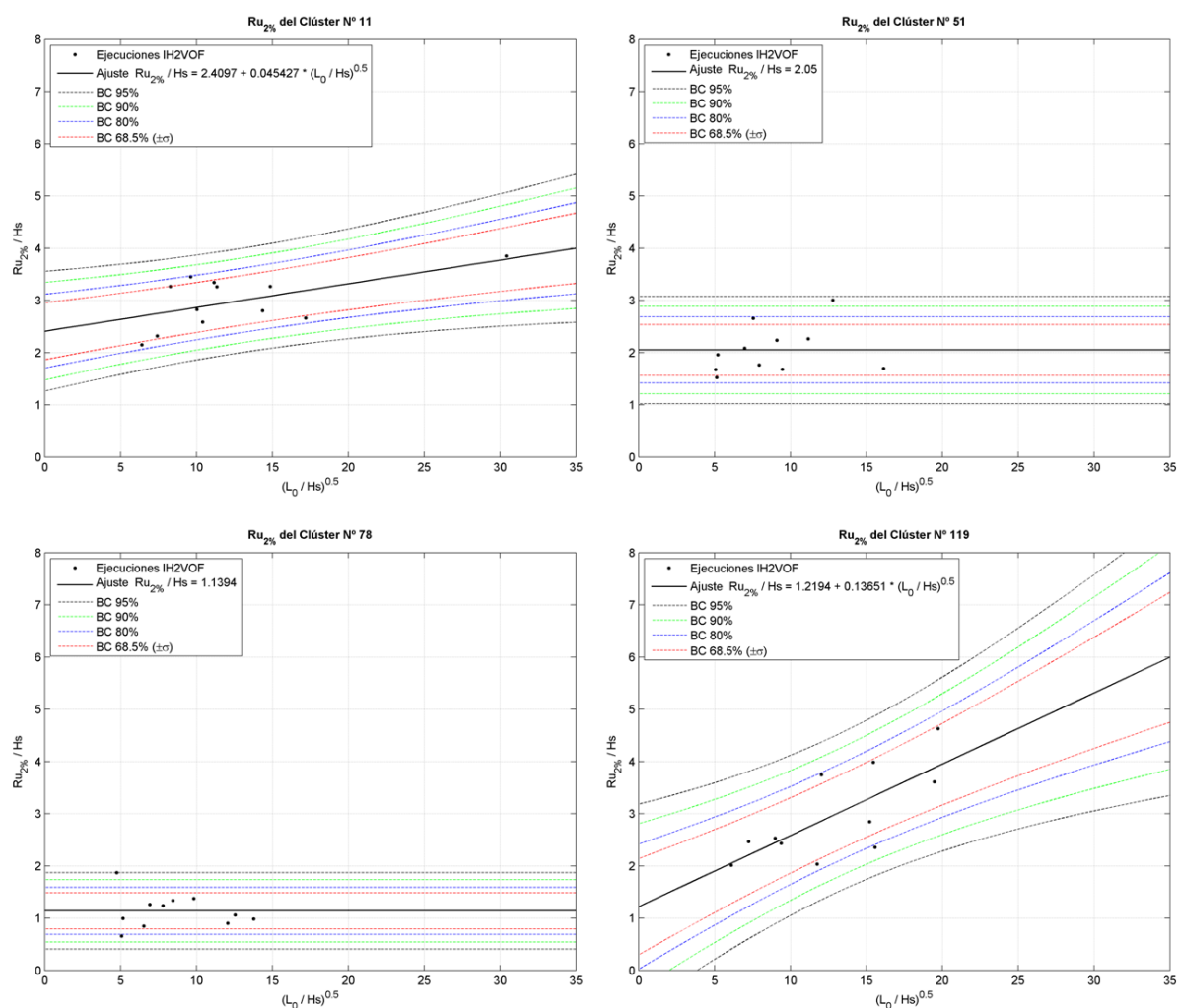
Figura 15. Ajustes lineales del run-up adimensional ( Ru_{2\%}/H_s ) en 4 clústers (Nº 11, 51, 78 y 119). Los puntos negros son los resultados de las ejecuciones del modelo IH2VOF, la línea negra es el ajuste de los datos a una recta y las líneas discontinuas son distintas bandas de confianza al 95%, 90%, 80% y 68.5% respectivamente.
