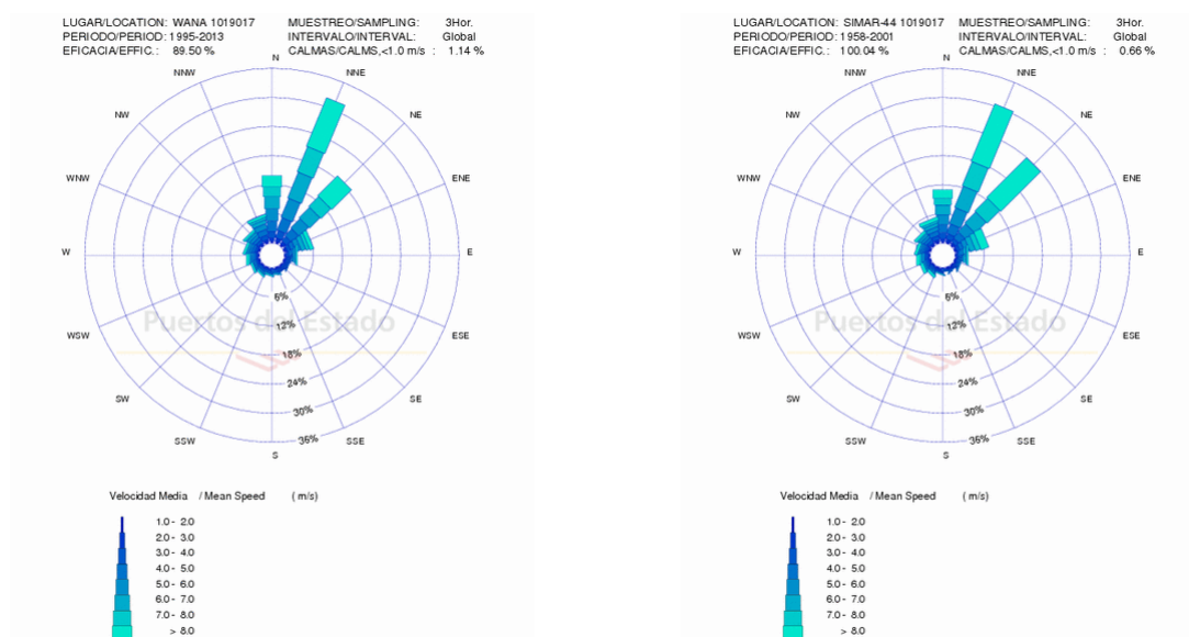
Figura 2. Rosa de vientos en un punto al norte de las Islas Canarias (WANA 1019017 y SIMAR-44 1019017), mostrando la predominancia de los vientos alisios (Fuente: Puertos del Estado)
