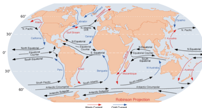
Figura 5. Corriente de Canarias. Zona oriental del giro subtropical del Atlántico Norte
